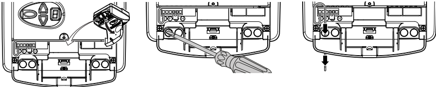
Kuva 8: Antennin asentaminen
