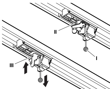
Rys. 16: Wysprzęglanie i zasprzęglanie napędu
