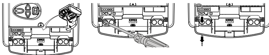
Fig. 8: Installera antennen
