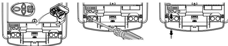
Rys. 8: Układanie anteny
