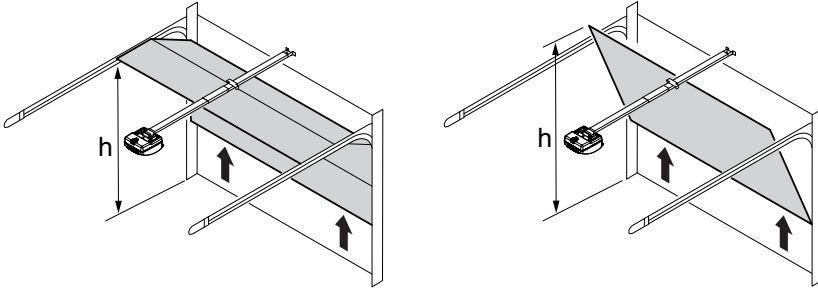
Kuva 5: Autotallinoven vapaan korkeuden mittaaminen
