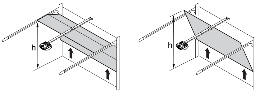
Obr. 5: Změřte světlostou výšku garážových vrat
