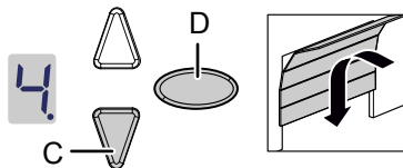
III. 13: Innstilling av endeveisposisjon LUKKE
